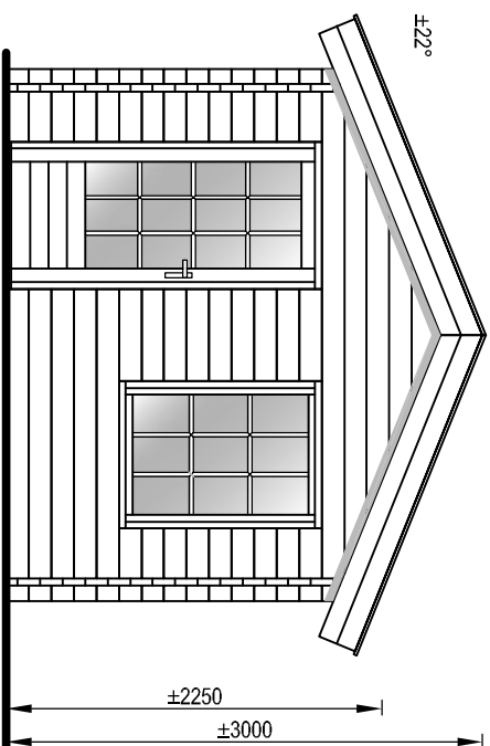
Voor aanzicht - Vorder Ansicht - Front view
