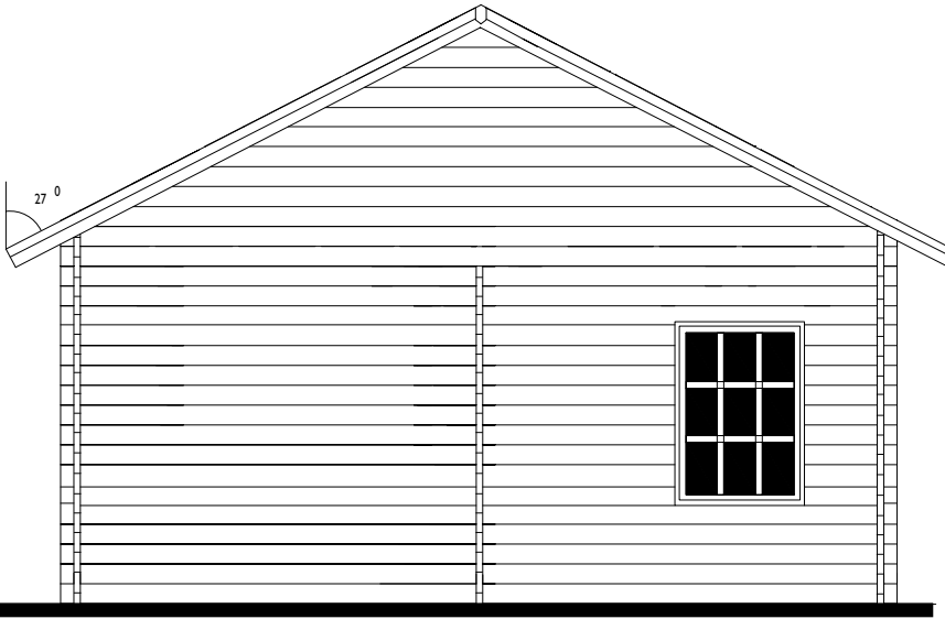
Achter aanzicht Hinten Ansicht Rear view
